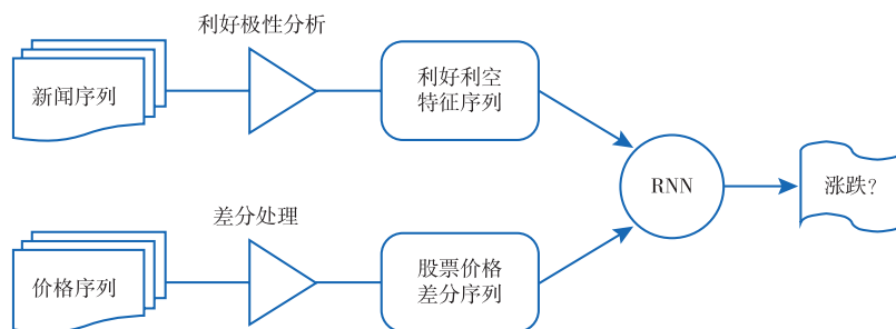
图 1 股票价格涨跌预测流程
