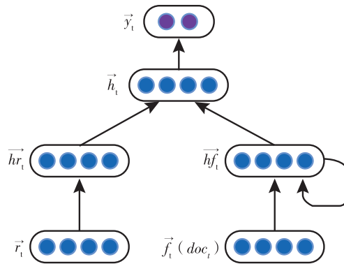
图2 循环神经网络预测
